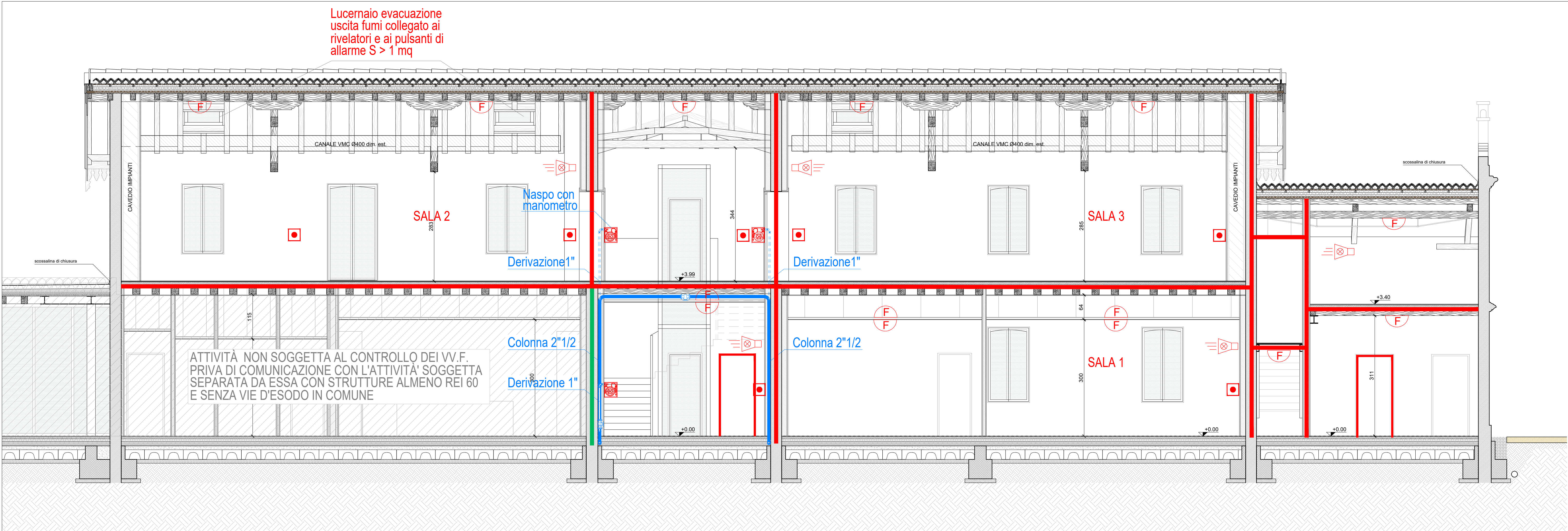
SEZIONE A-A - scala 1:50
