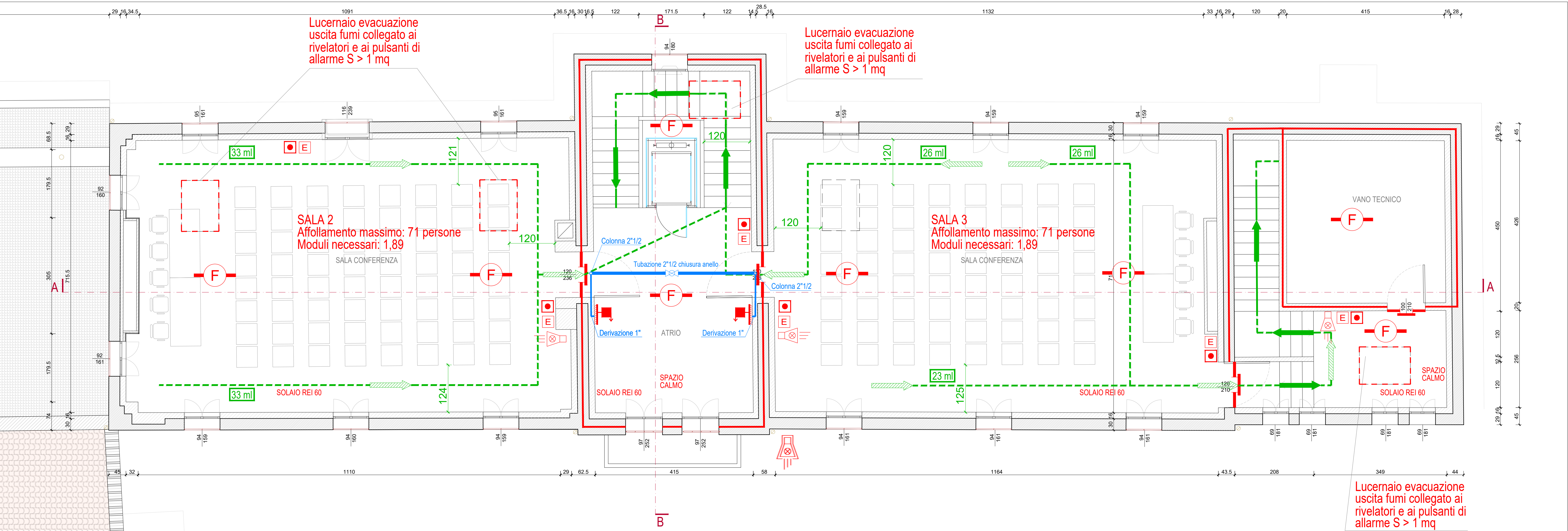
PIANTA PIANO PRIMO - scala 1:50
