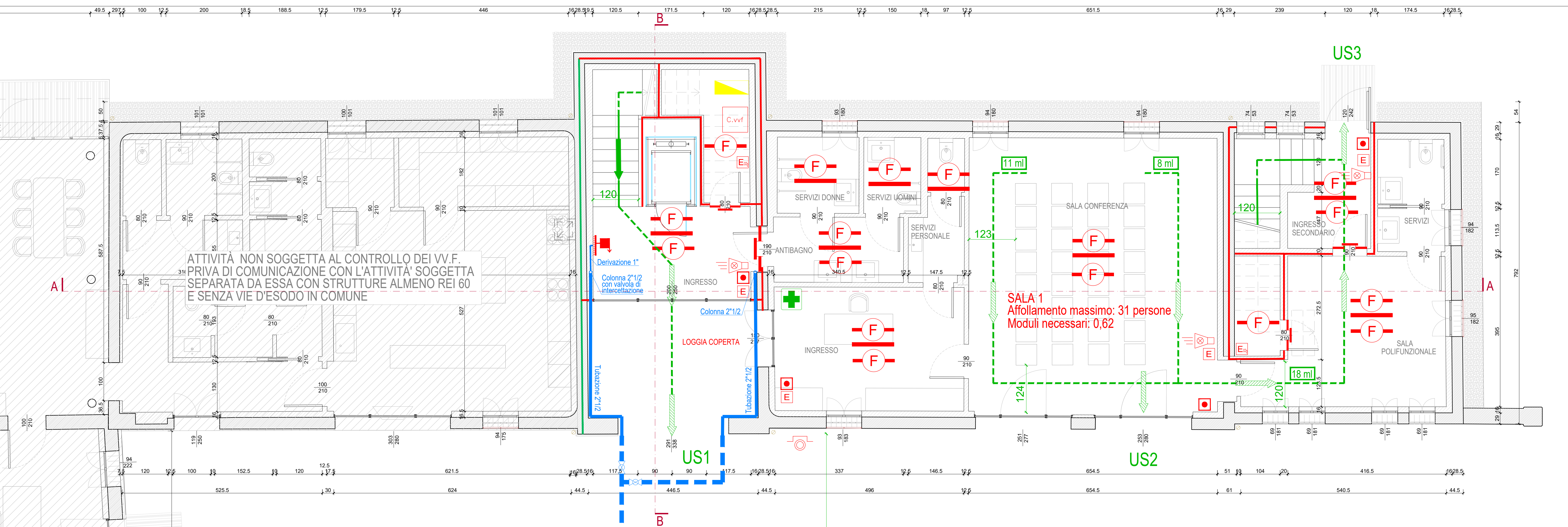
PIANTA PIANO TERRA - scala 1:50
