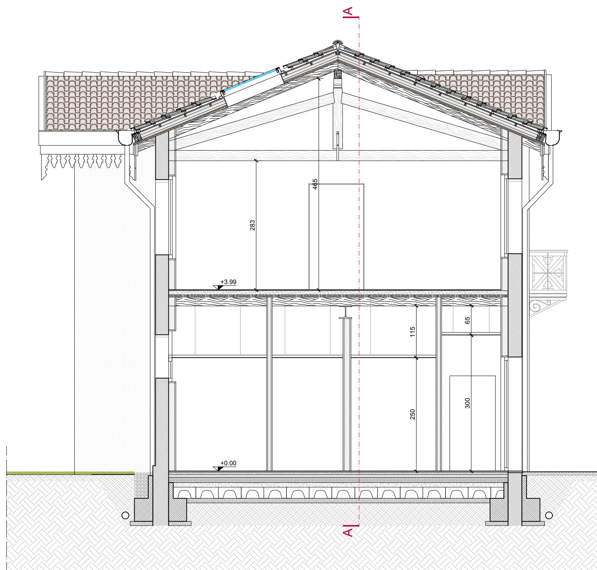
SEZIONE BB
