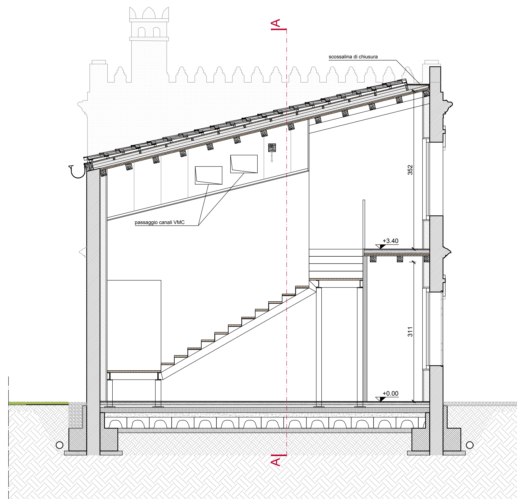
SEZIONE DD
