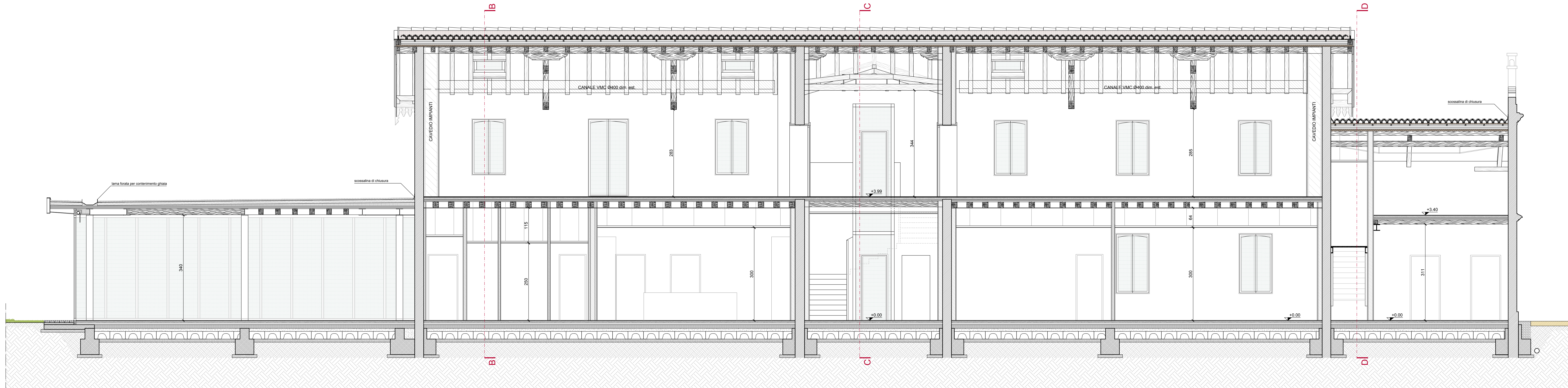
SEZIONE AA
