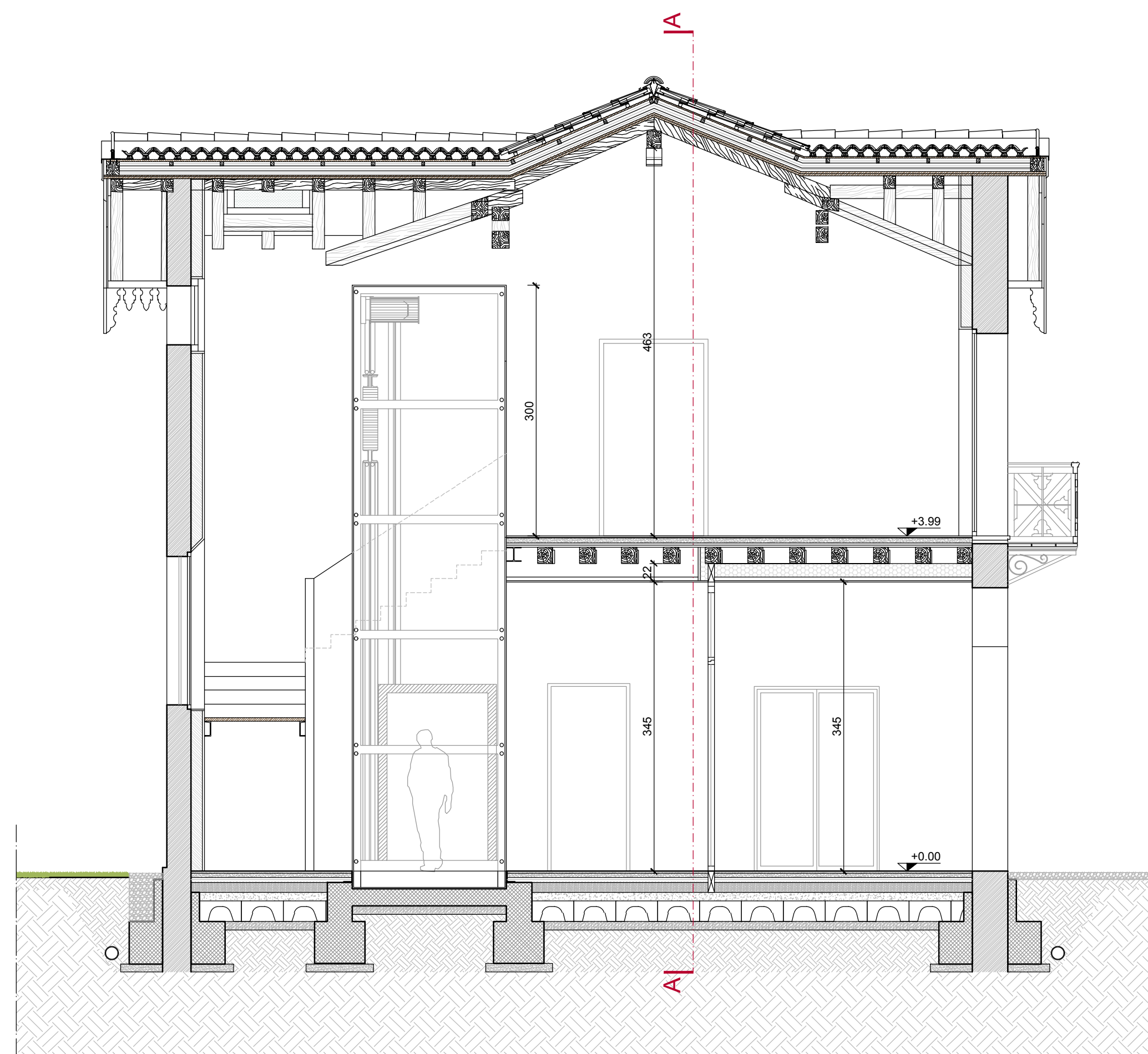
SEZIONE CC
