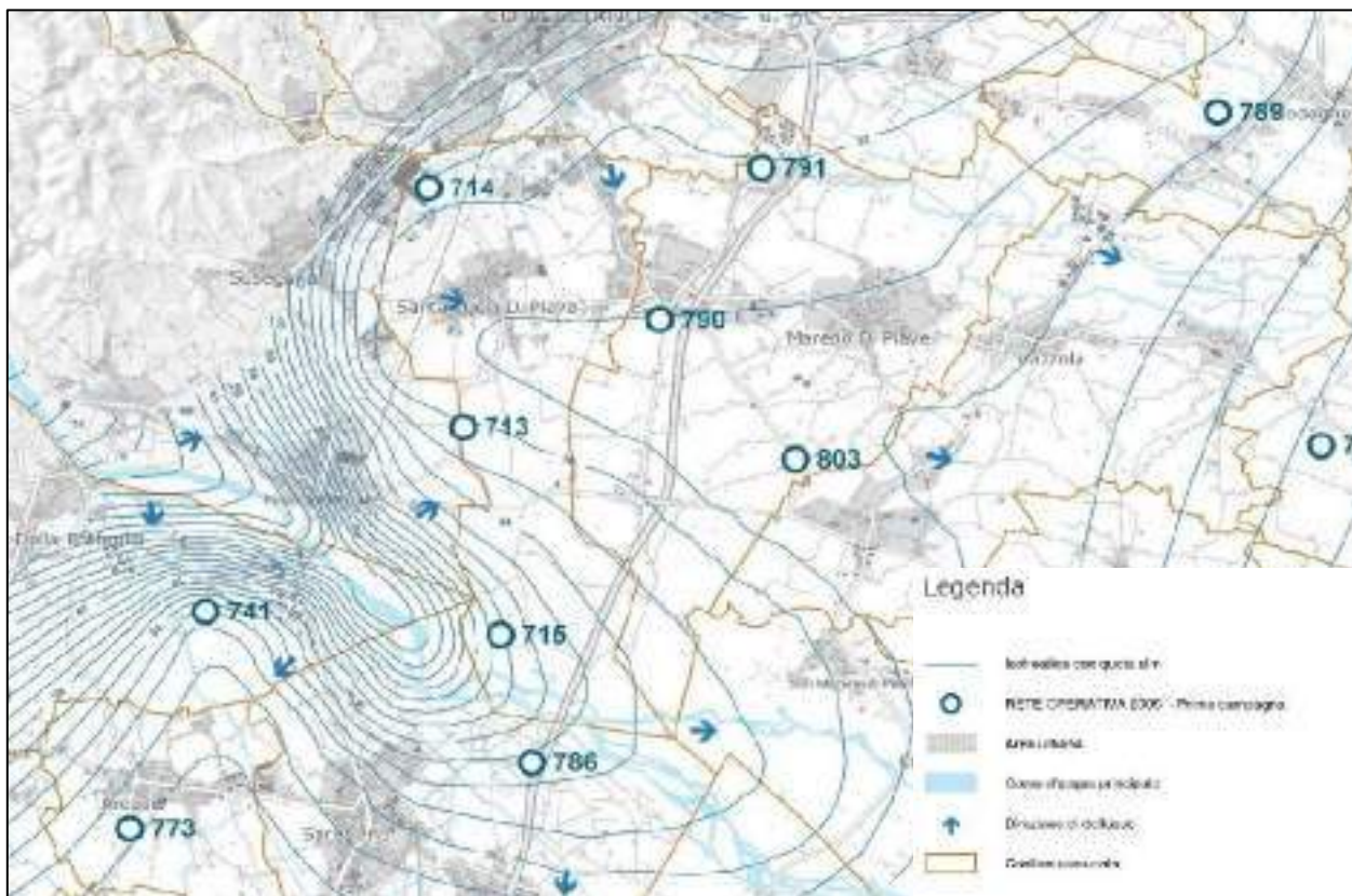
Stralcio della Carta freaticometrica provinciale - deflussi di magra del 2002
