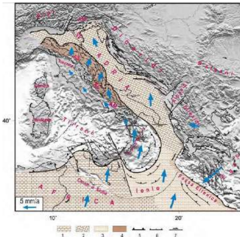
Schema tettonico della penisola italiana. Legenda: 1- Placca Africana con crosta continentale; 2- Microplacca Adria con crosta continentale; 3- Area di transizione tra Placca Africana e Microplacca Adria; 4- Catena Appenninica (AS: Appennino Settentrionale; AC: Appennino Centrale; AM: Appennino Meridionale); 5- Fronte della catena Appenninica; 6- Faglie normali; 7- Faglie trascorrenti (SV: Linea Schio-Vicenza); ASE: Alpi Meridionali Orientali. La lunghezza della freccia blue è proporzionale alla velocità di movimento della placca.
